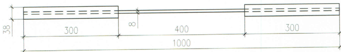
Слика 1: Графички приказ испитиваних узорака (димензије дате у mm)
